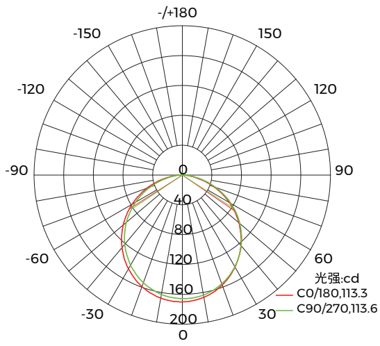
配光曲线
